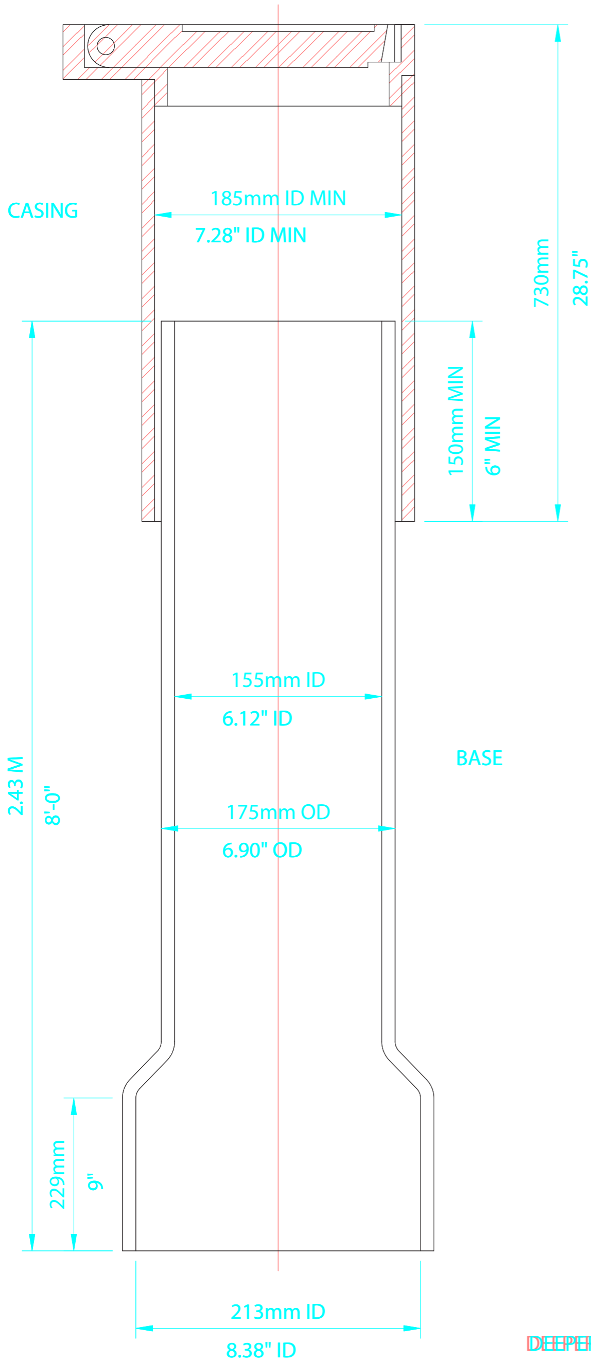
SECTION A-A
